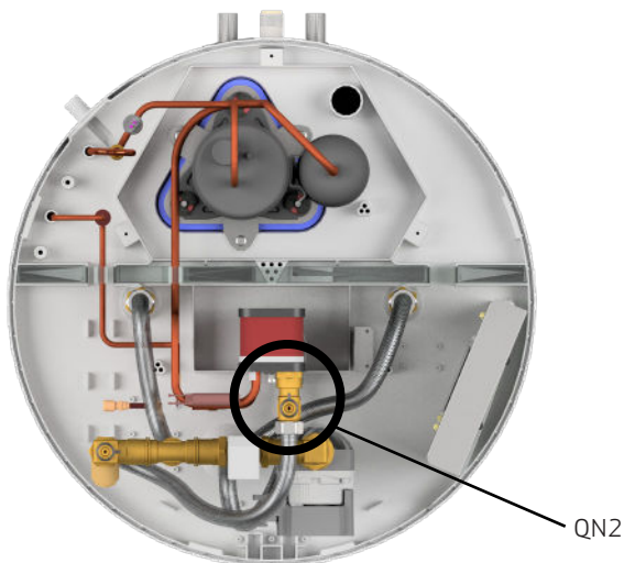
Afbeelding 14 - Plaats van de ontlufter (zie omcirkeld).
