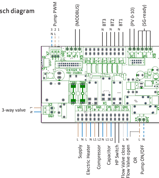
Afbeelding 13 - Elektrische schema
